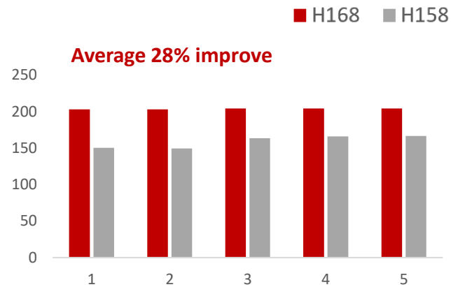
SA UL Performance
